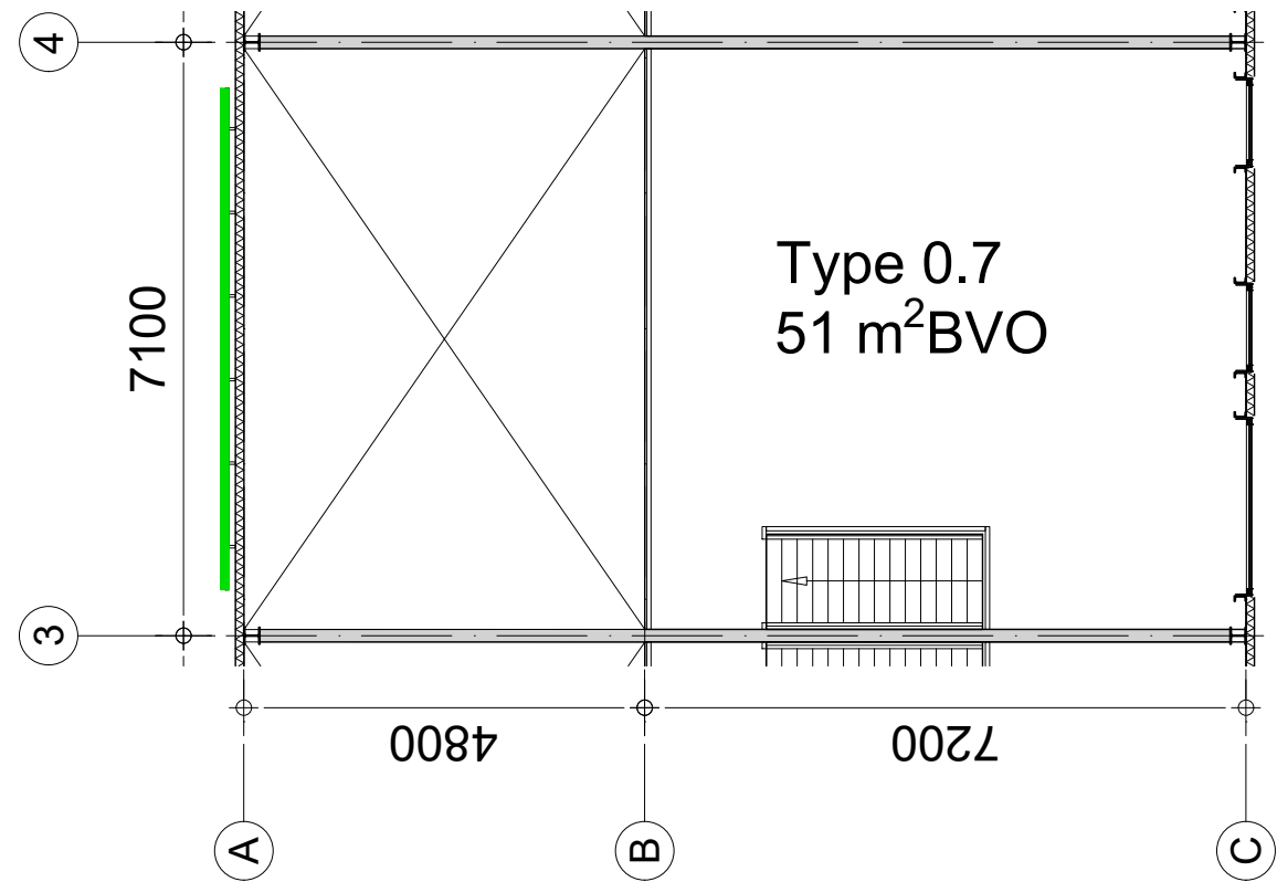
Eerste verdieping
