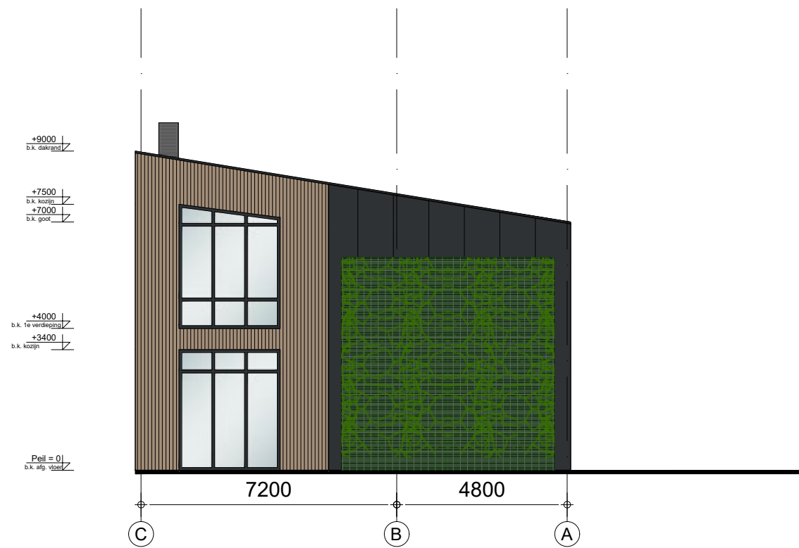
Rechter zijgevel
