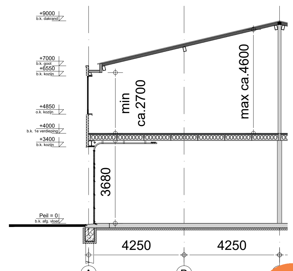
Doorsnede
