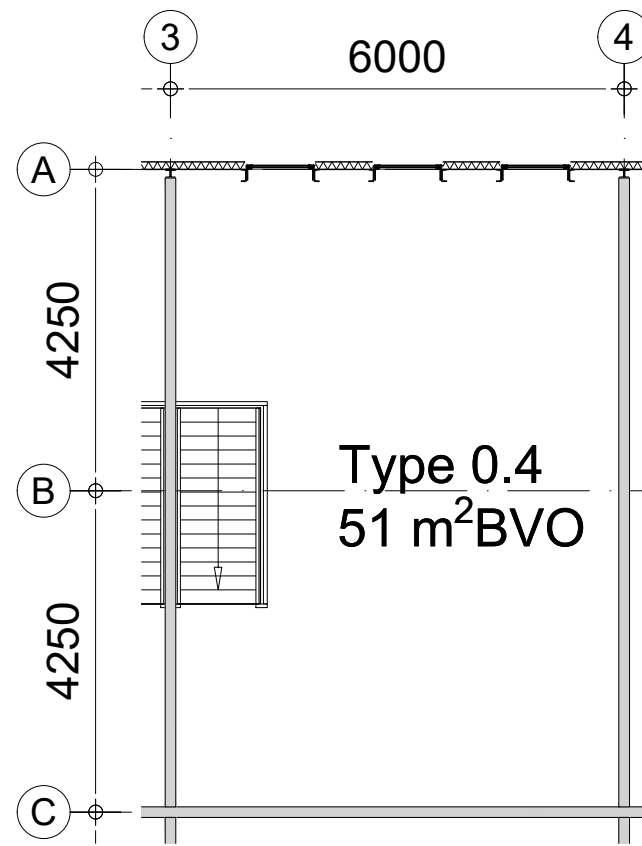
1e Verdieping
