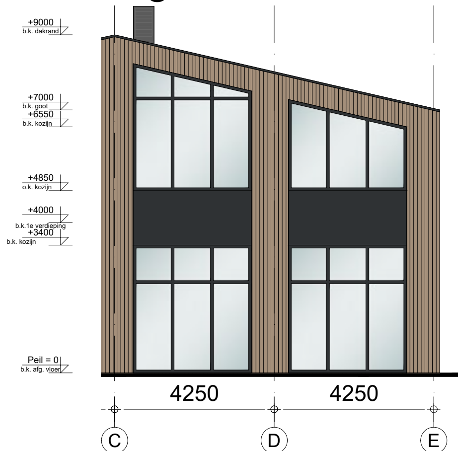
Voorgevel
