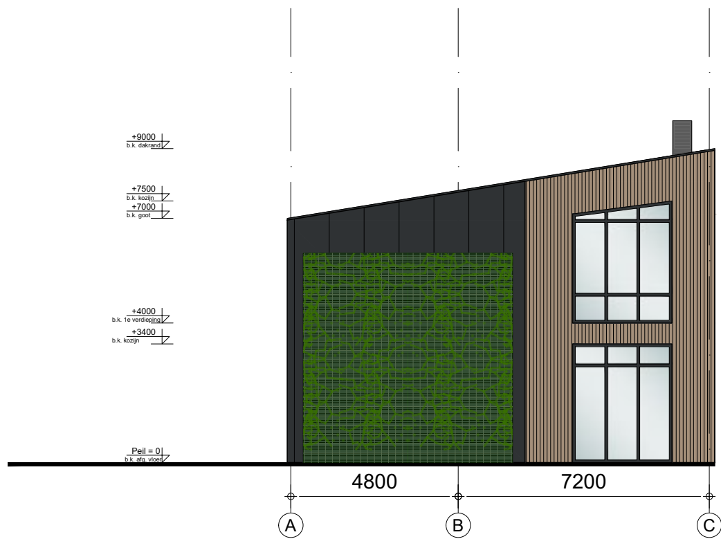
Linker zijgevel
