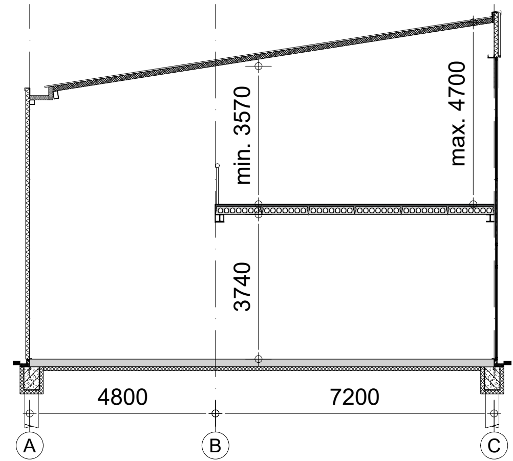
Doorsnede
