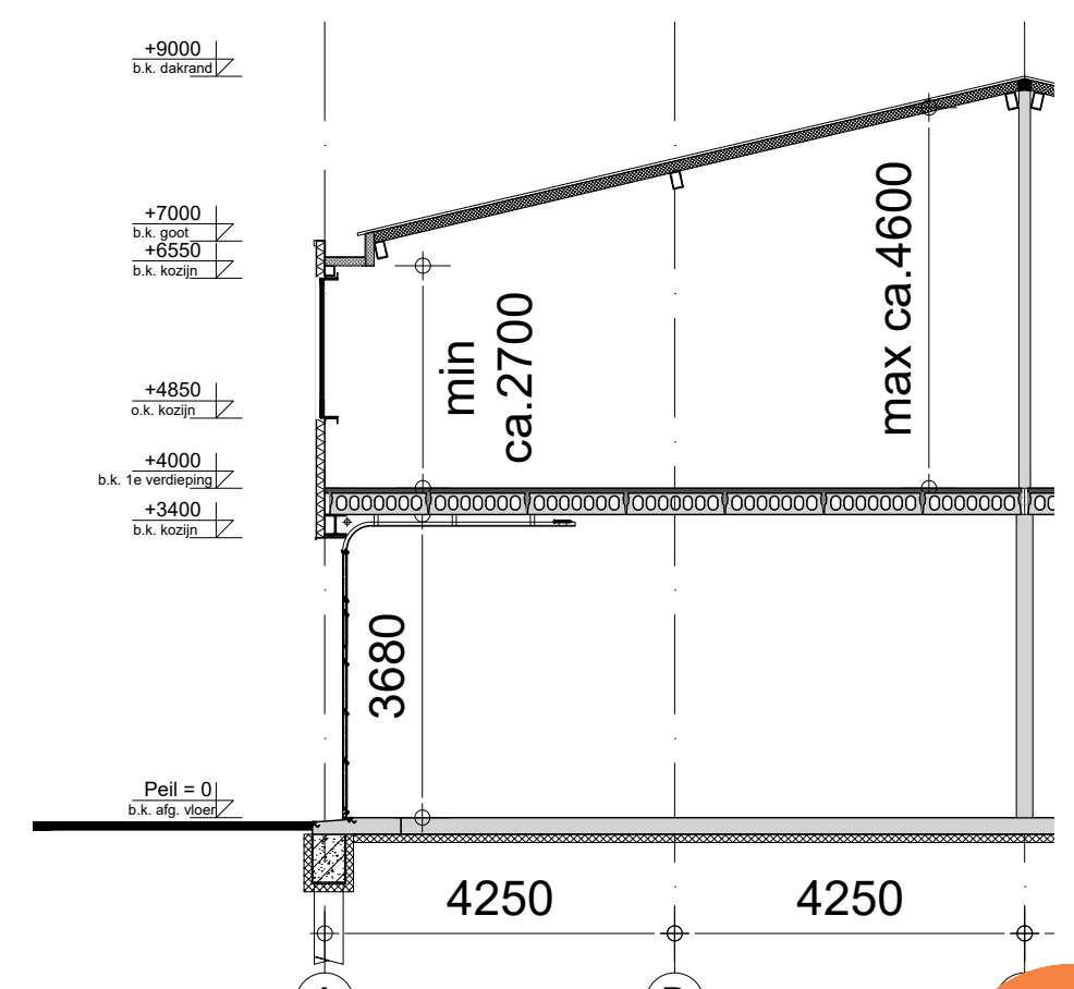
Doorsnede
