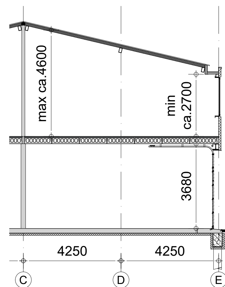
Doorsnede
