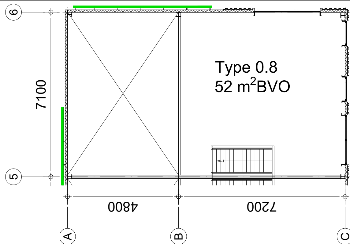
Eerste verdieping
