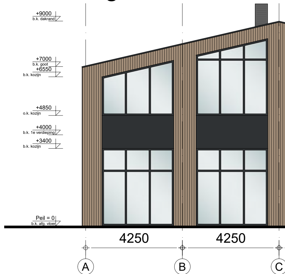
Voorgevel
