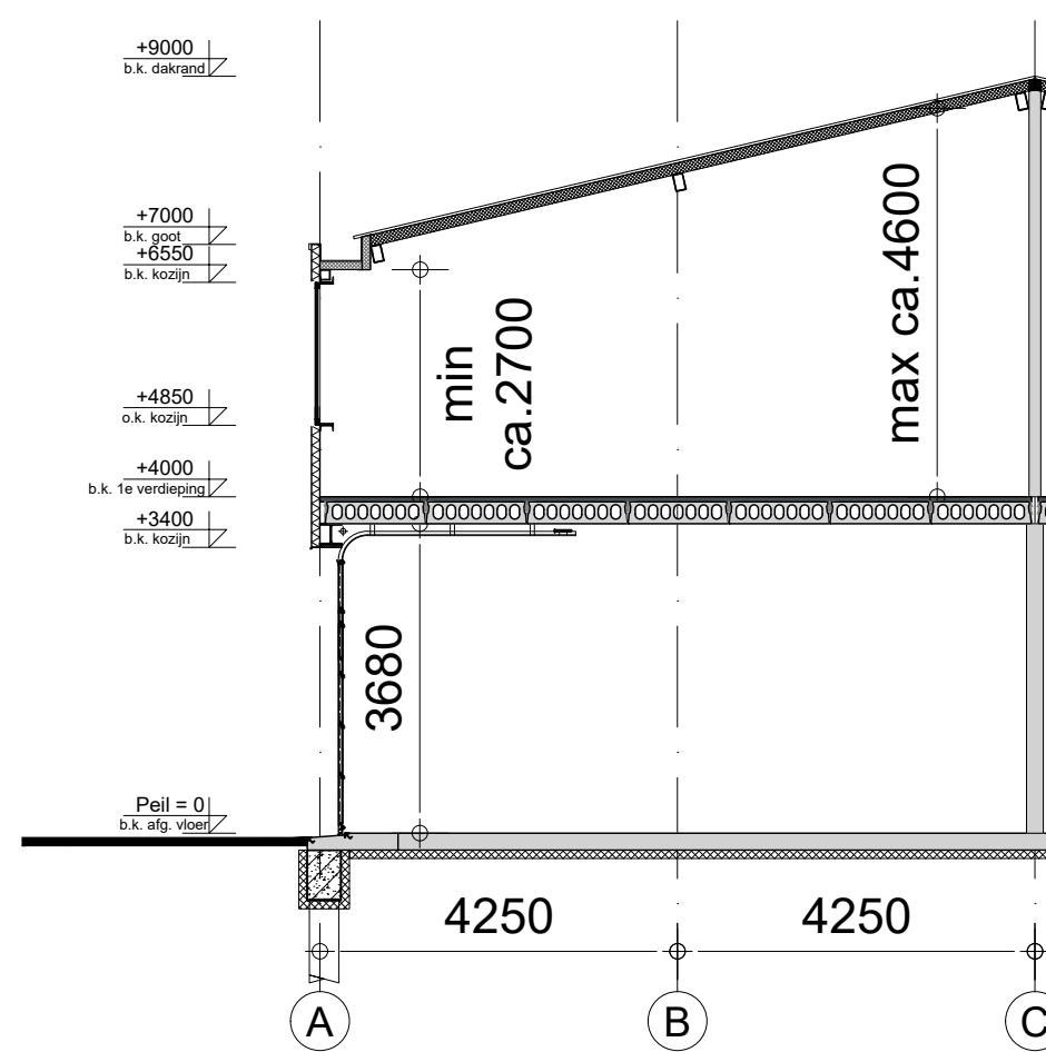
Doorsnede
