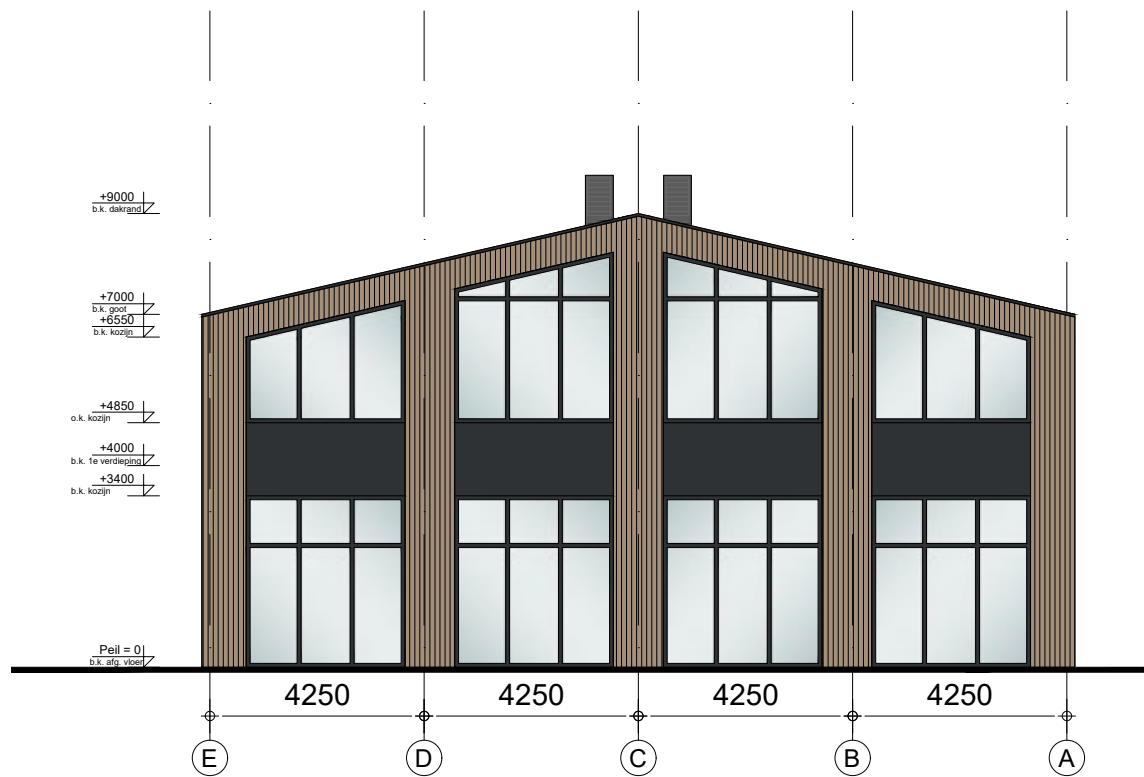
Voorgevel
