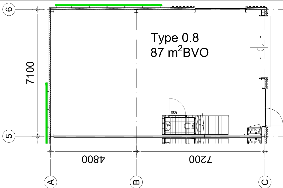
Begane Grond
