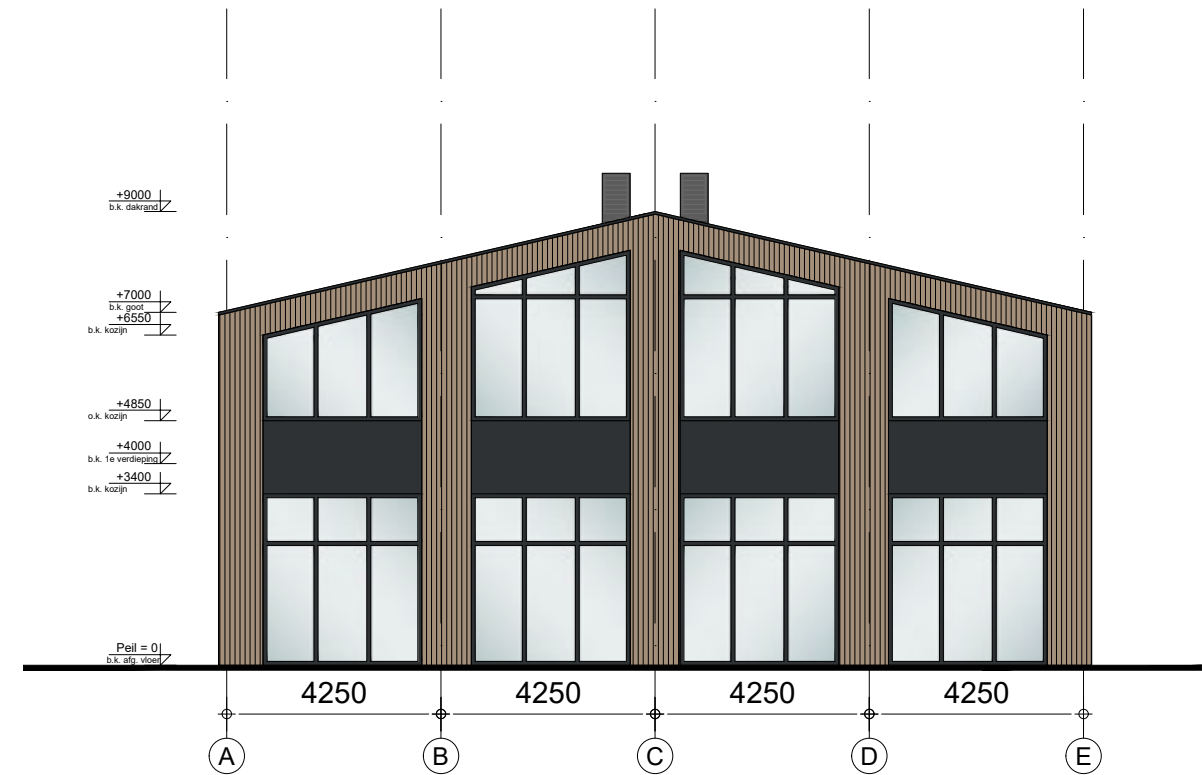
Achtergevel
