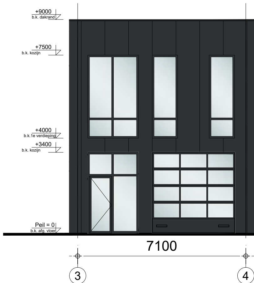
Voorgevel
