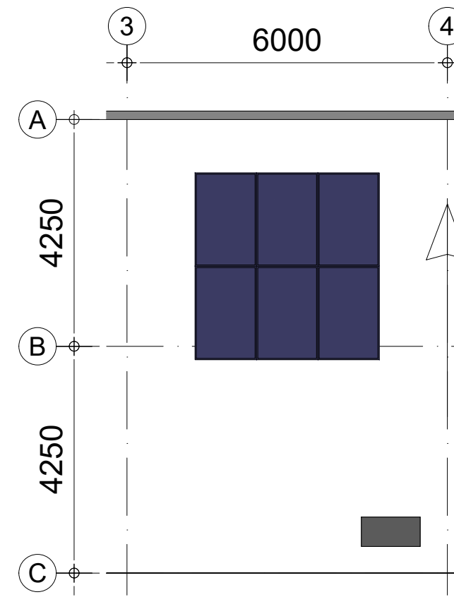
Dakoverzicht
