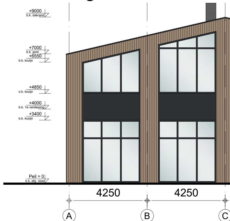
Voorgevel
