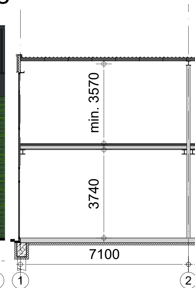
Doorsnede
