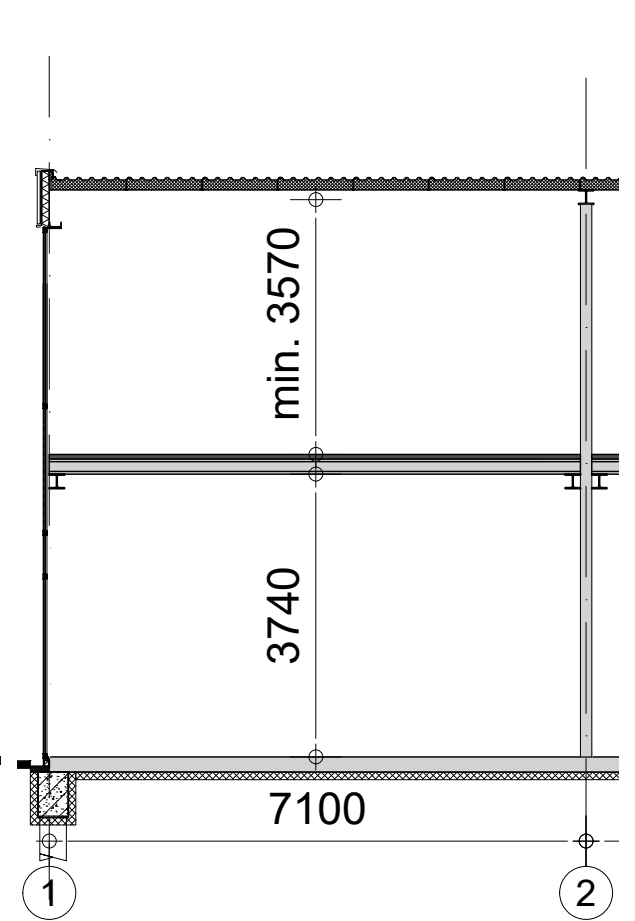
Doorsnede
