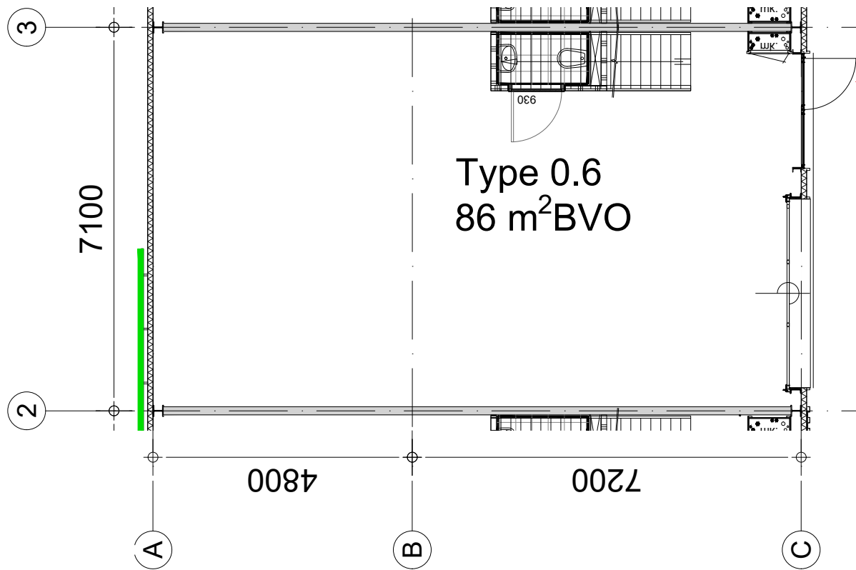
Begane Grond
