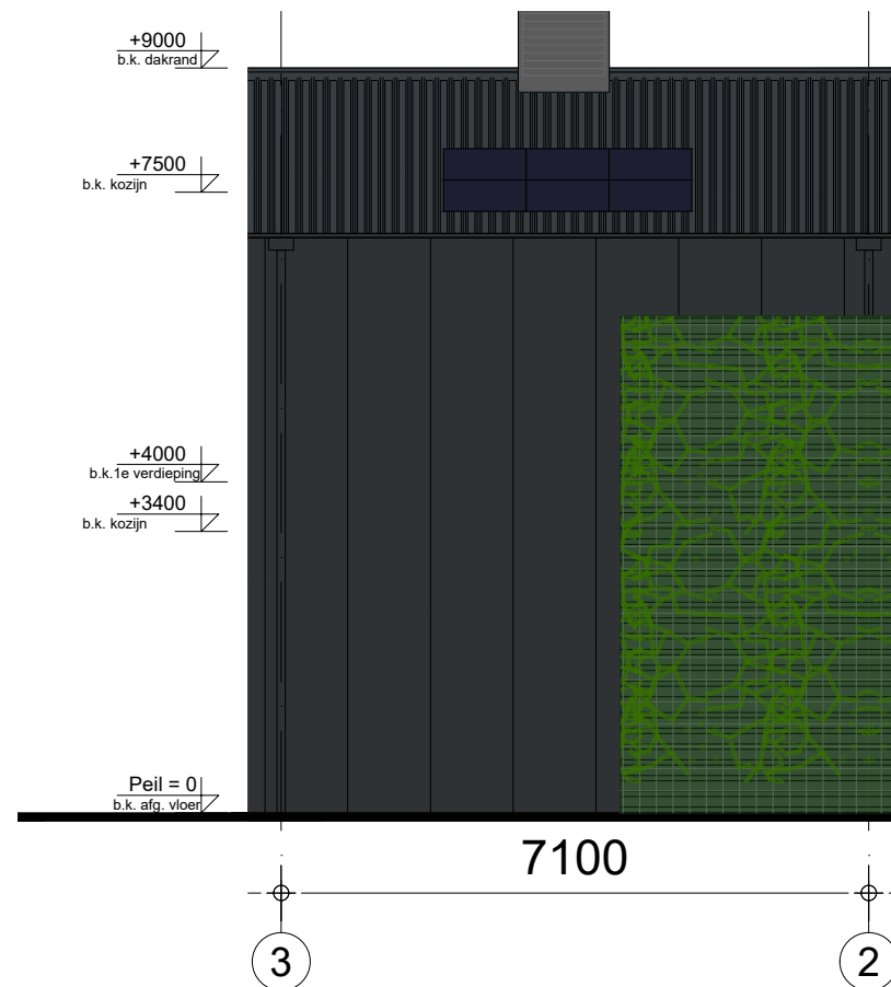
Achtergevel
