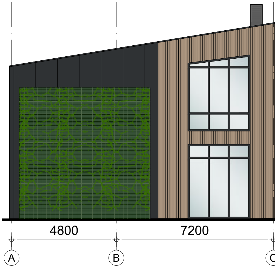
Zijgevel
