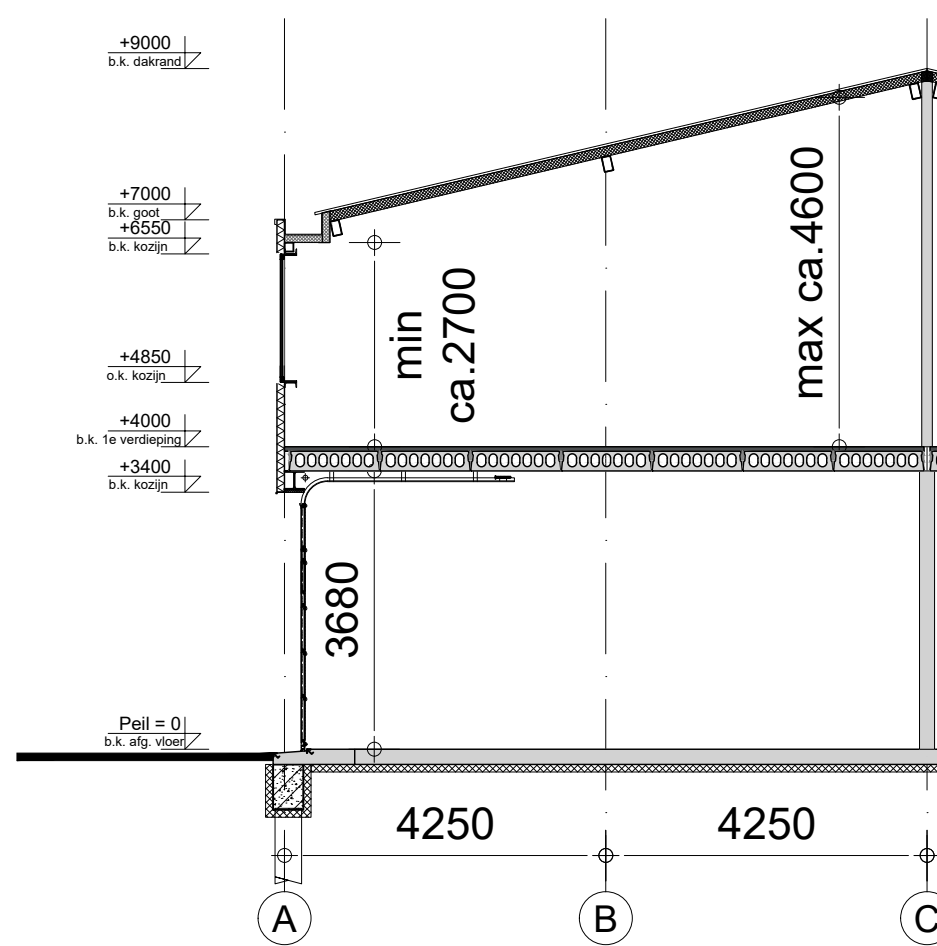
Doorsnede
